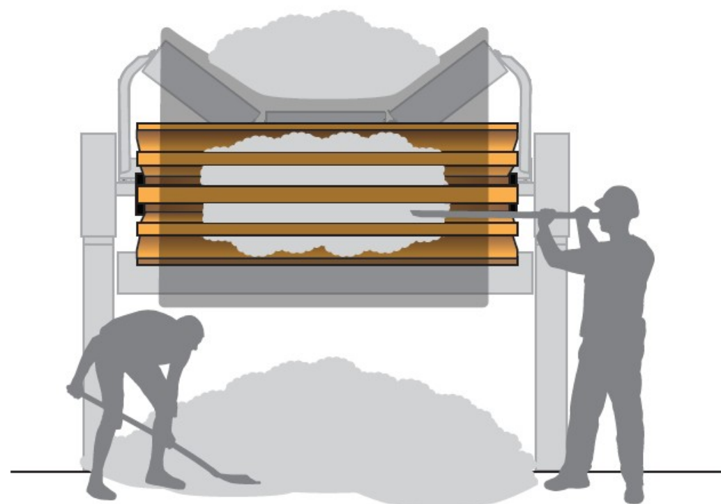
Tambor Wing Tradicional
