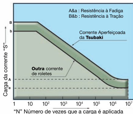
Curva S-N
