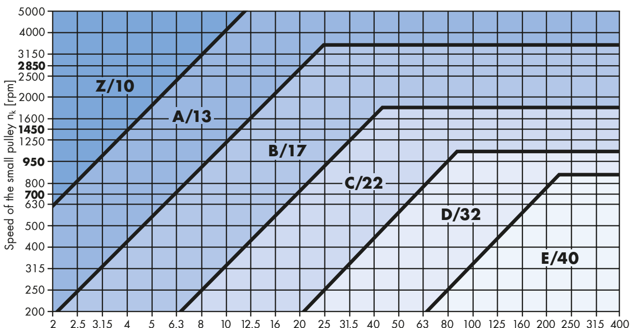
Diagram 1: optibelt VB classic V-belts DIN 2215
