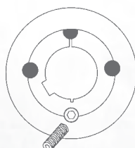
Dimensions TB 1008-3030
