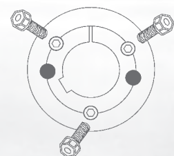
Dimensions TB 3525-5050
