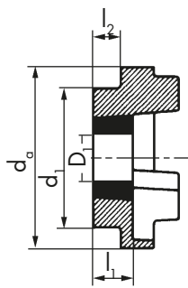
F flange
