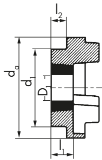
H flange
