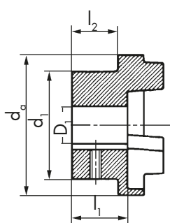
B flange
