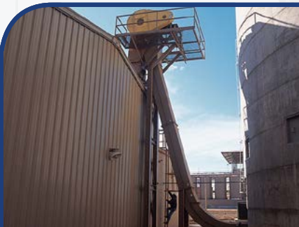
Transportador de Corrente Tipo "L"
