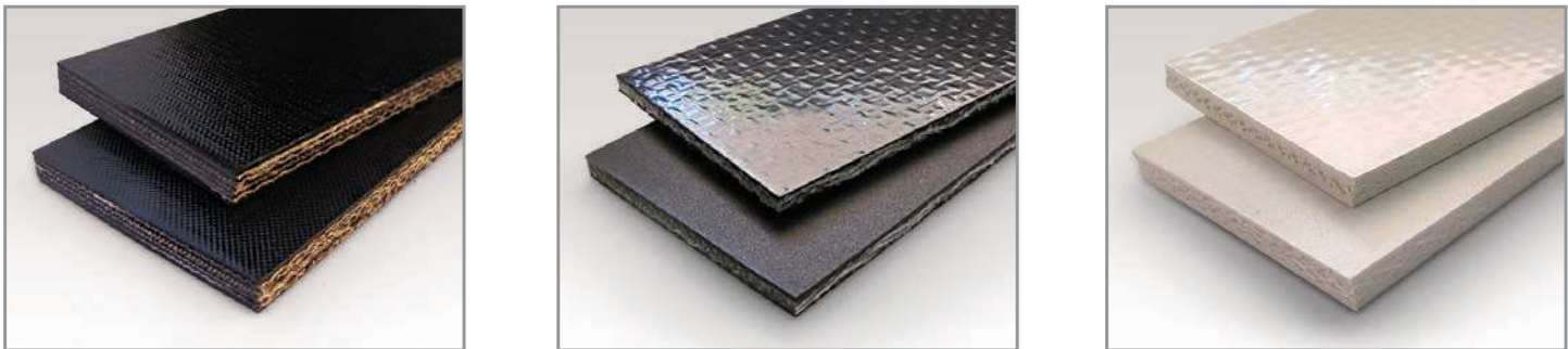
BORRACHA (Premium) 3/330, 4/440, 3/600, 4/800 (Padrão) 220, 330, 440, 600, 800 PVC (padrão) 200, 250, 350, 450, 600 PVC (alimentos e grãos) 200, 350, 400 Branco e preto. Também disponível em Branco FDA
